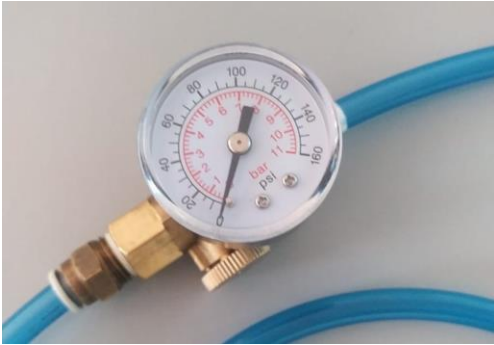
Fig. 12: Válvula ajustadora de aire con manómetro
