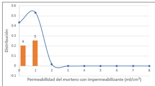
Fig. 13. Gráfica de distribución normal con los resultados de la prueba de permeabilidad a especímenes de mortero con impermeabilizante.
