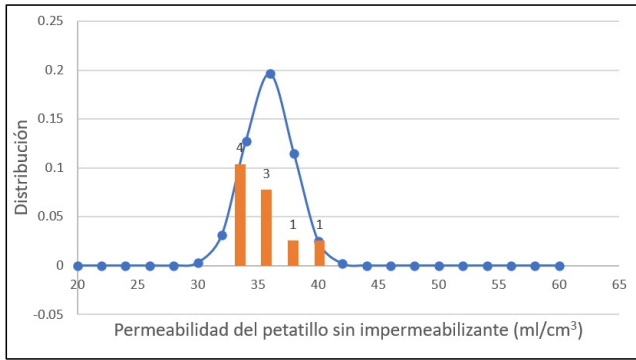
Fig. 14. Gráfica de distribución normal con los resultados de la prueba de permeabilidad a especímenes de petatillo sin impermeabilizante.
