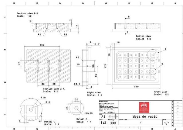
Fig. 7. Dibujo 2D de la mesa de vacío.
