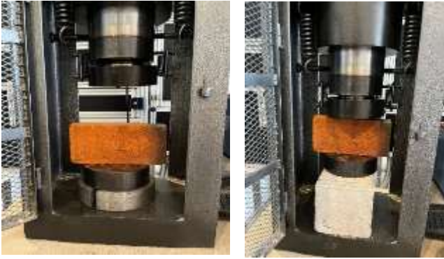
Fig. 1: Posición del ladrillo en la prensa hidráulica.
