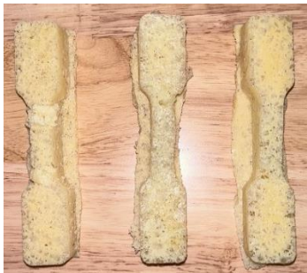
Fig. 3. Probetas de espuma Ibero prueba de tensión. Fuente: elaboración propia.
