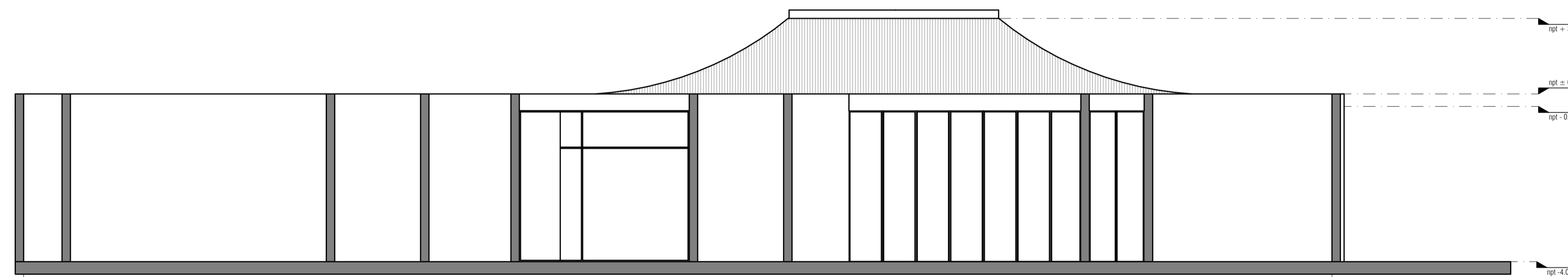
FACHADA OESTE - EDIFICIO 1 NIVEL -2.70
