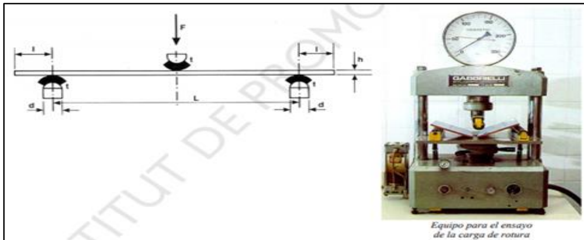
Figura 37 - Equipo de laboratorio para el cálculo de resistencia. Fuente (IPC, 2015)
