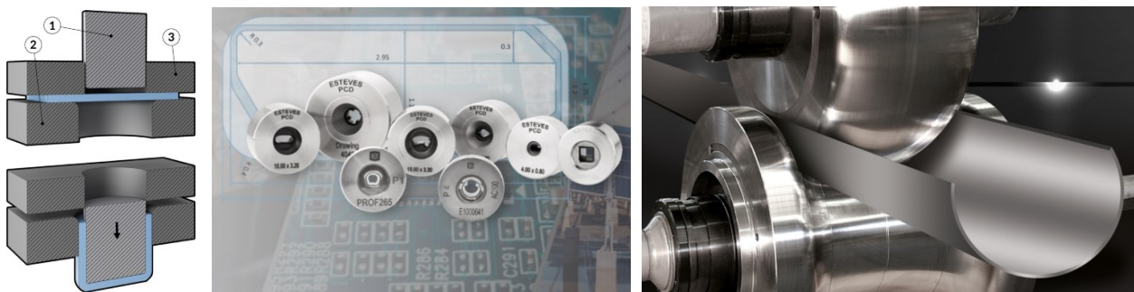
Figura 13. Proceso de formado: embutido profundo [31], dados con forma para extruido en frío [32], de un tubo con costura con proceso de rodado [33]
