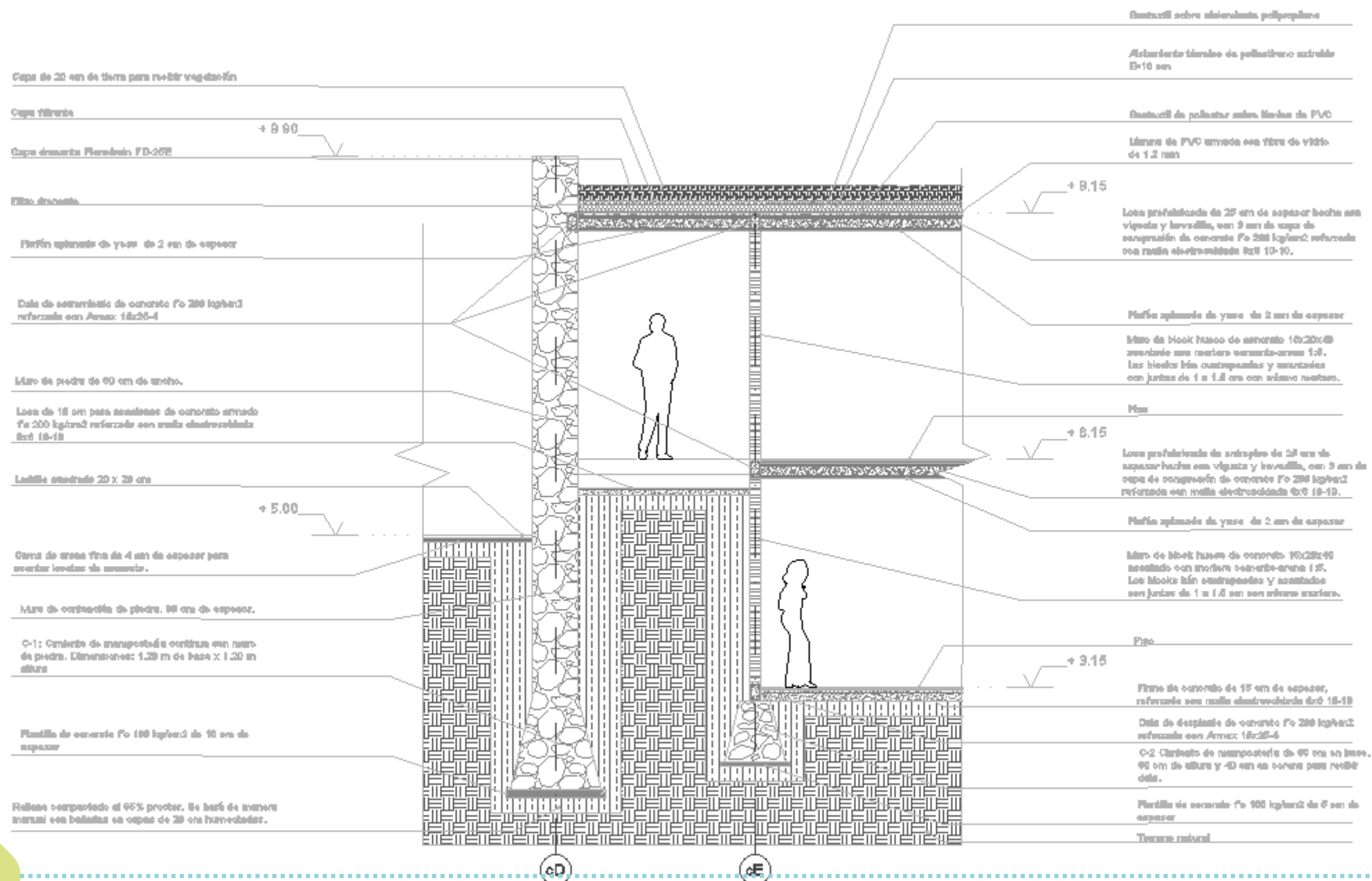
Corte por Fachada Y-Y' Esc: 1:25
