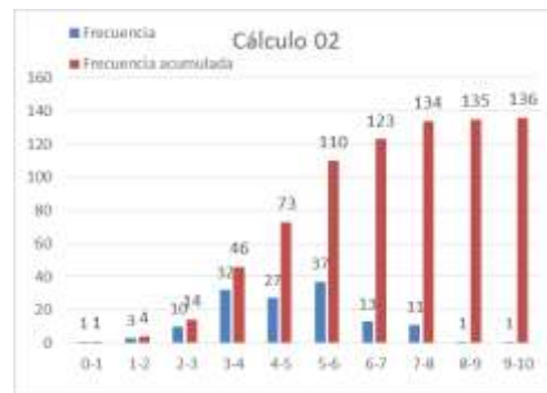
Fig. 2. Distribución de las frecuencias Cálculo 02.
