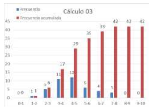
Fig. 3. Distribución de las frecuencias Cálculo 03.
