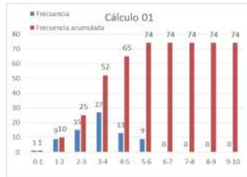
Fig. 1. Distribución de las frecuencias Cálculo 01.
