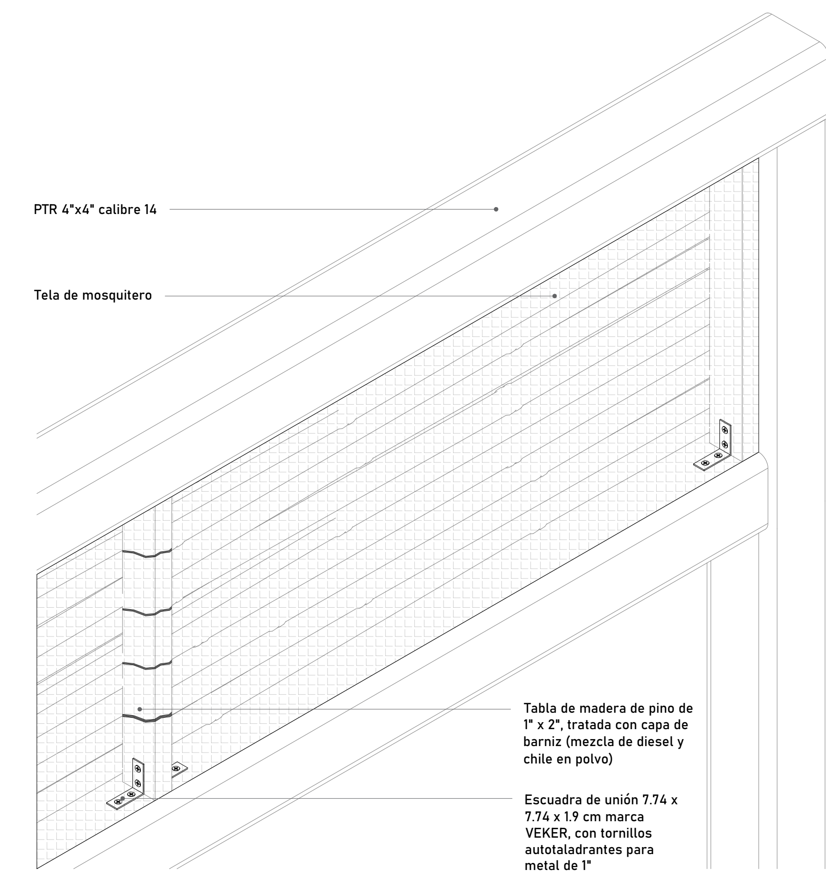
Detalle en isométrico
