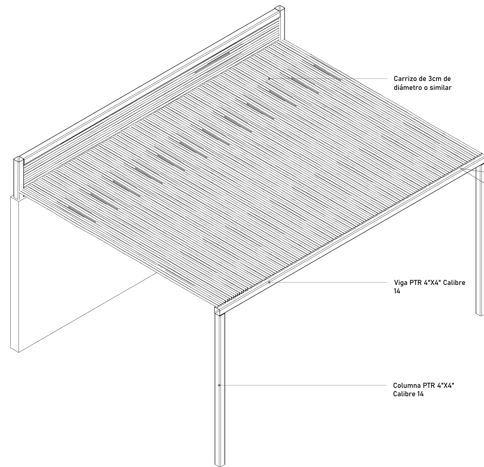
Isométrico de módulo tipo
