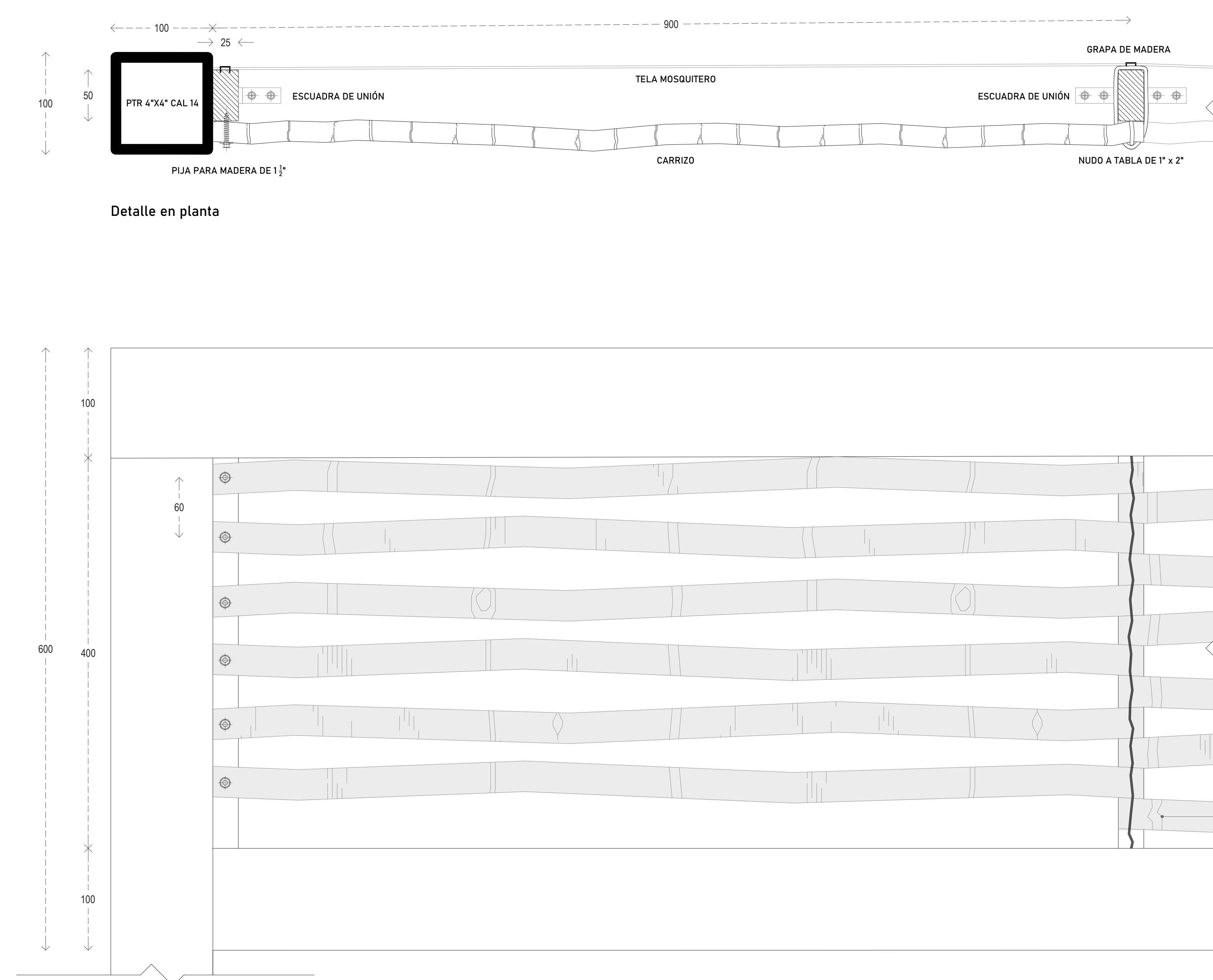
Detalle en alzado
