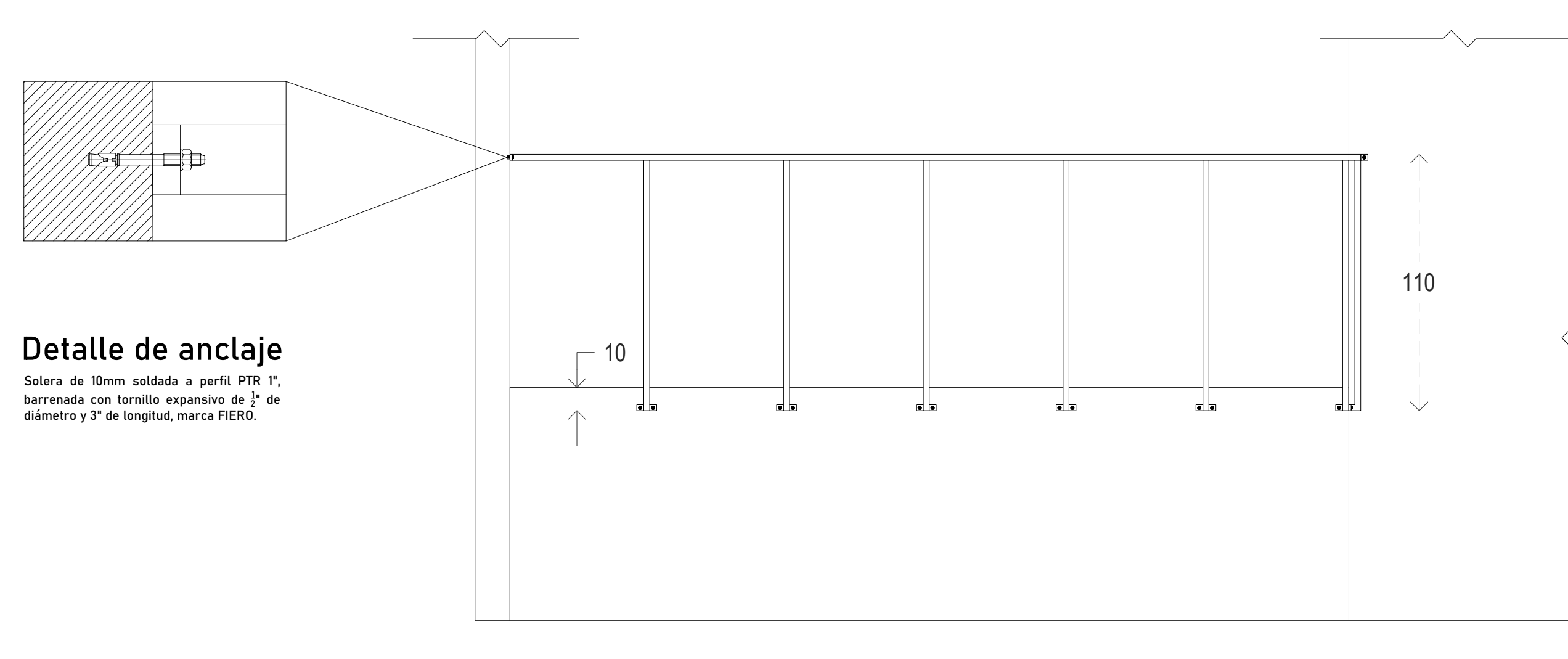
Alzado frontal
