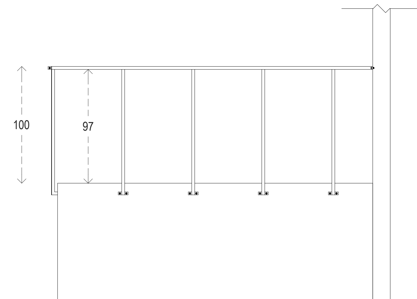
Alzado lateral
