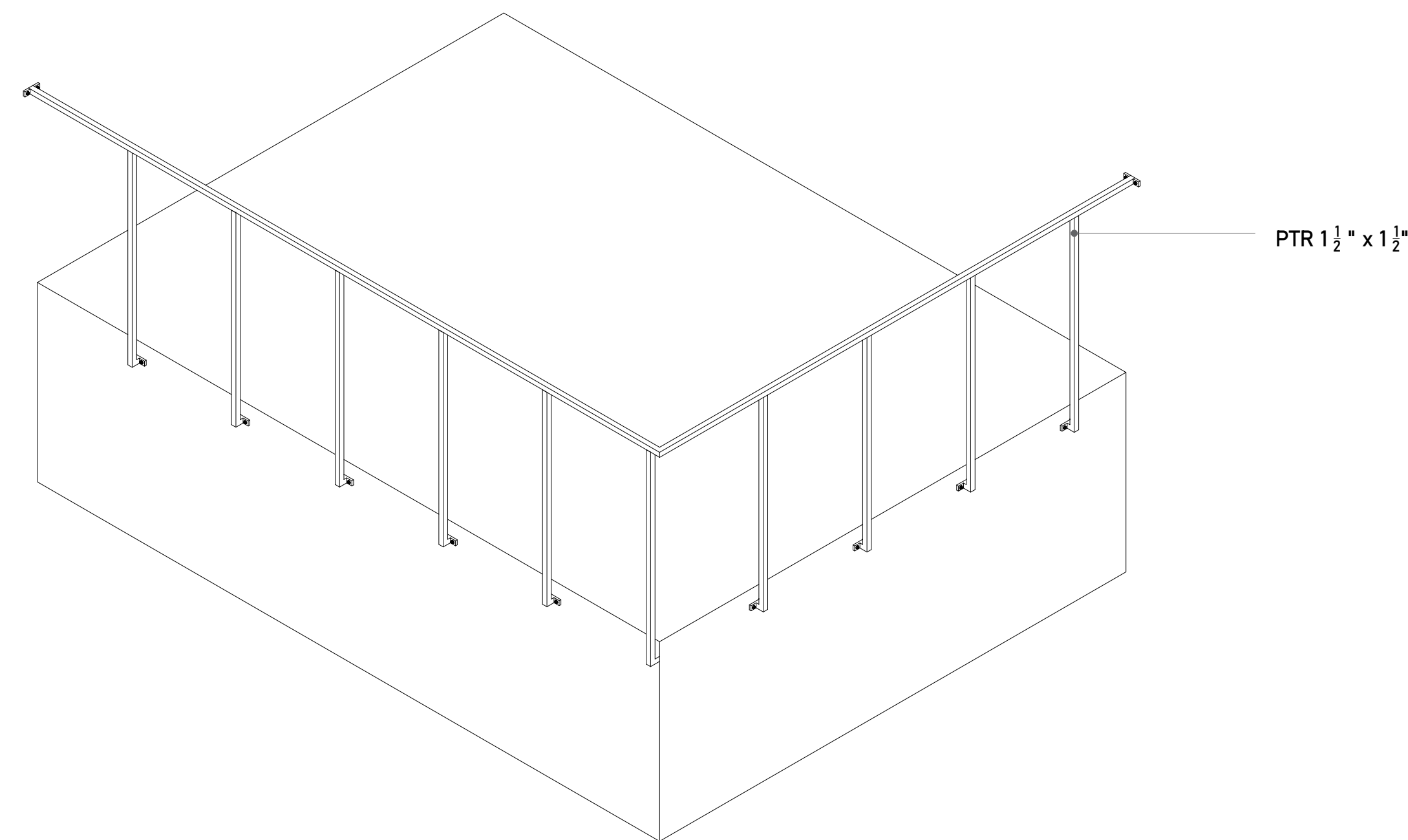
Isométrico
