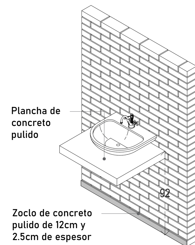
Isométrico
