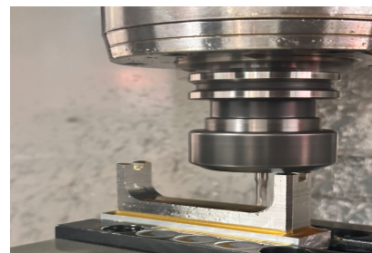
Fig. 10 Unión en Fresa Haas CNC.
