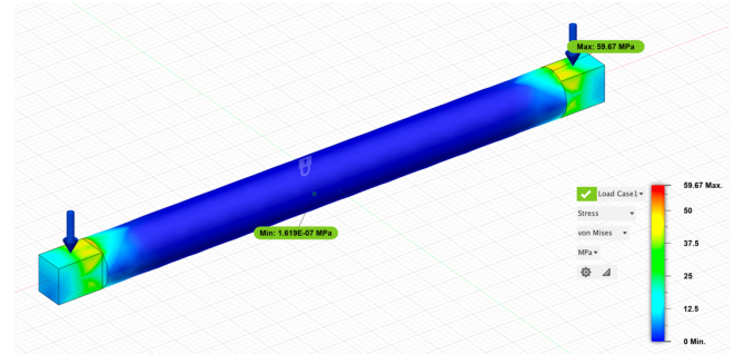
Fig. 14 Análisis de elementos finitos de Ele con 1000 N en Fusion.
