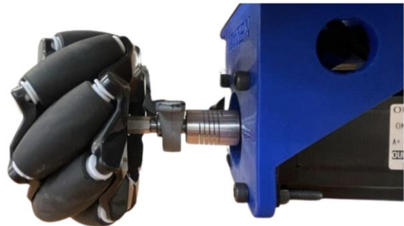
Fig. 6. Acoplamiento motor-eje-llanta.
