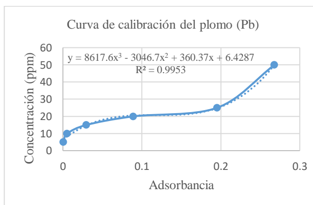
Fig. 6: Gráfica de curva de calibración de la adsorbancia contra la concentración del plomo (Pb).
