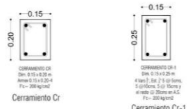
Cerramiento Cr-1
