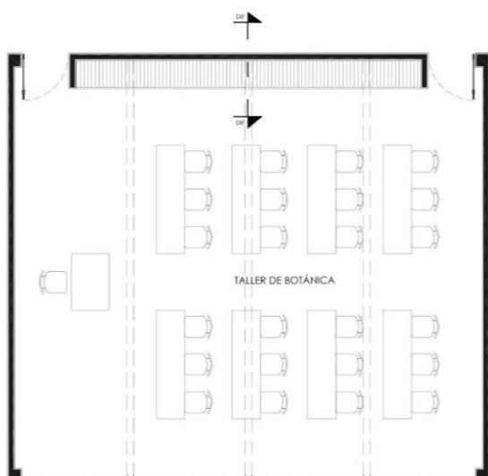
Planta arquitectónica
