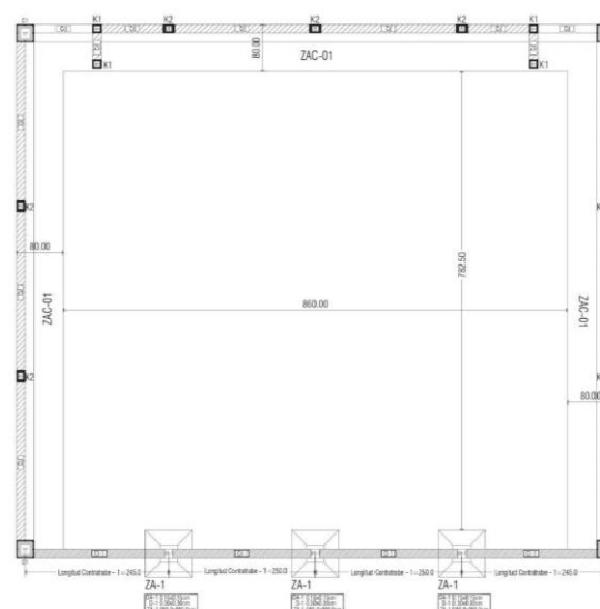
Planta cimentación
