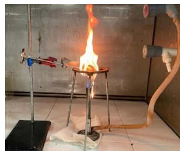
Fig. 17. Prueba de combustión espuma Ibero. Fuente: elaboración propia.
