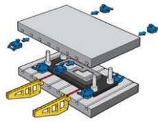
Ilustración 15 ejemplo de modelado de elementos SMED. Referencia en Bibliografía
