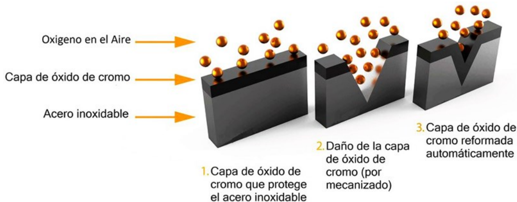
Figura 2. Capa pasivada del acero inoxidable [4]
