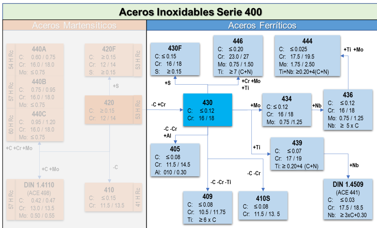
Figura 7. Aceros Ferríticos [11]
