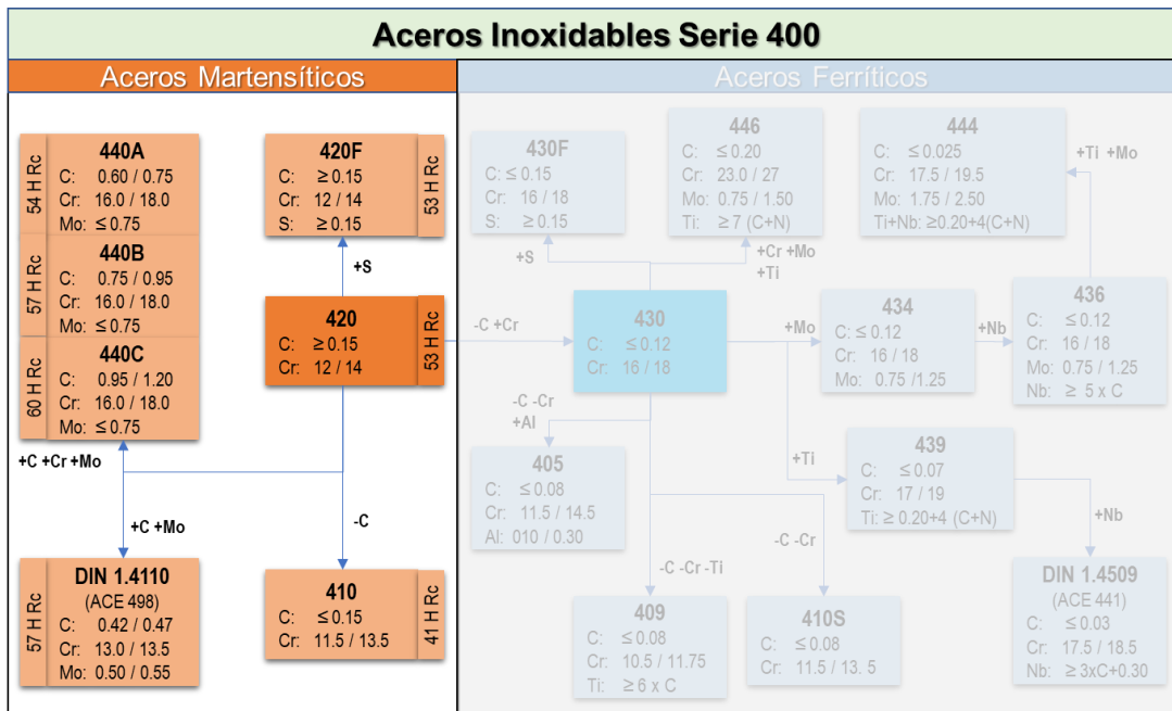
Figura 5. Aceros Martensíticos [11]
