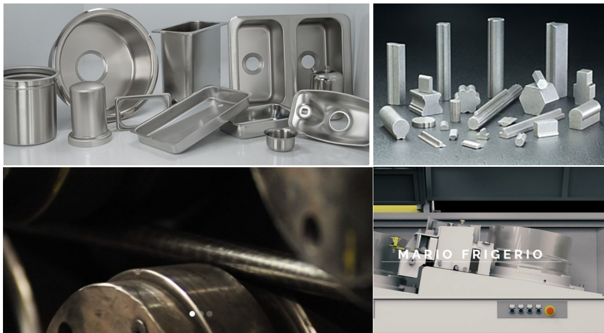
Figura 14. Proceso de formado: partes formadas mediante un embutido profundo e hidro formado [34] , perfiles con formas especiales fabricados mediante extruido en frío [35] , formado en frío de una barra [36] , sección de una máquina para trefilado de alambre [37]
