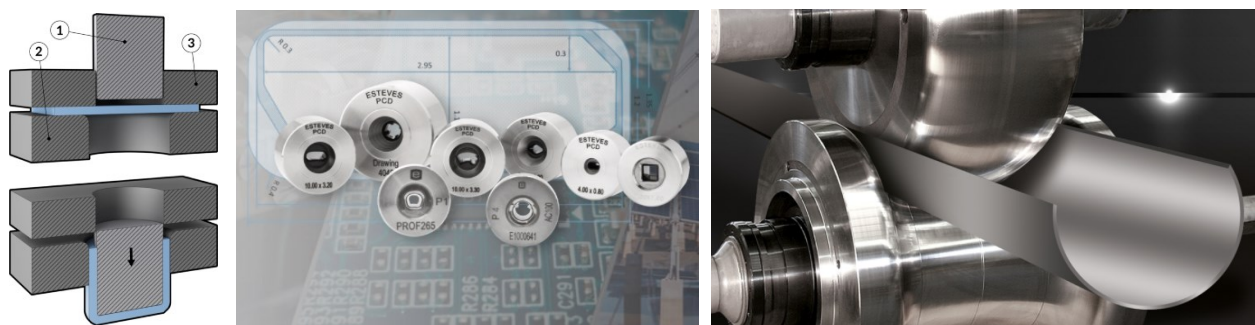
Figura 13. Proceso de formado: embutido profundo [31], dados con forma para extruido en frío [32], de un tubo con costura con proceso de rolado [33]
