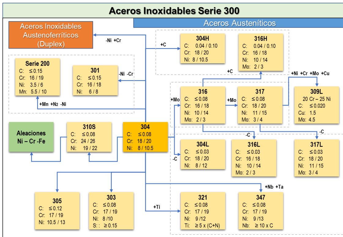
Figura 9. Aceros Austeníticos [11]
