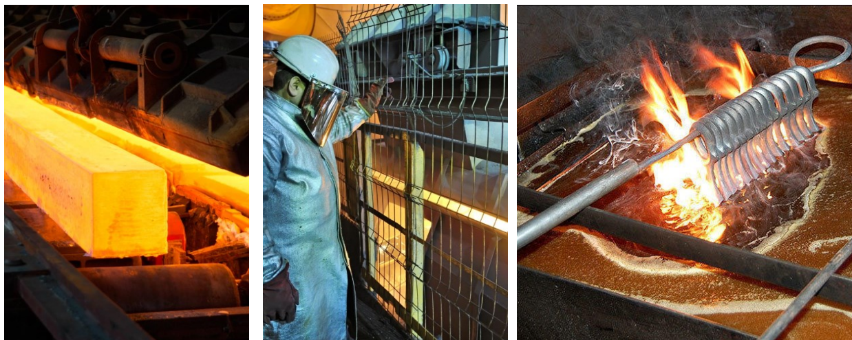
Figura 18. Tratamientos térmicos de aceros: temple y revenido [44] , temple por inducción [45] , templado en aceite [46]
