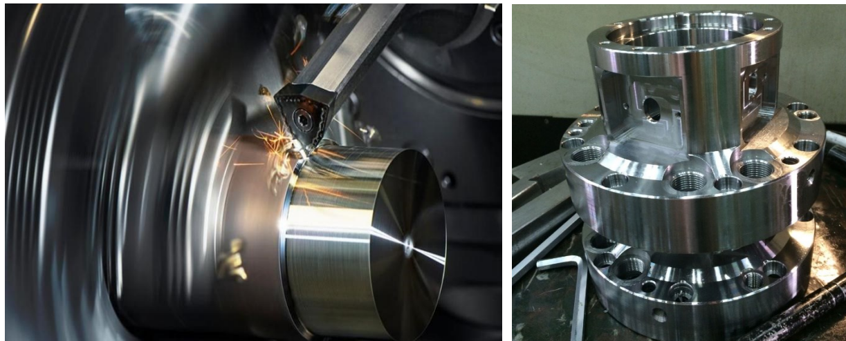
Figura 17. Procesos de maquinado: torneado de una barra de acero inoxidable [42], fresado complejo por control numérico [43]
