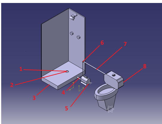
Figura 1. Sistema integrado de la casa de ejemplo, mostrando
