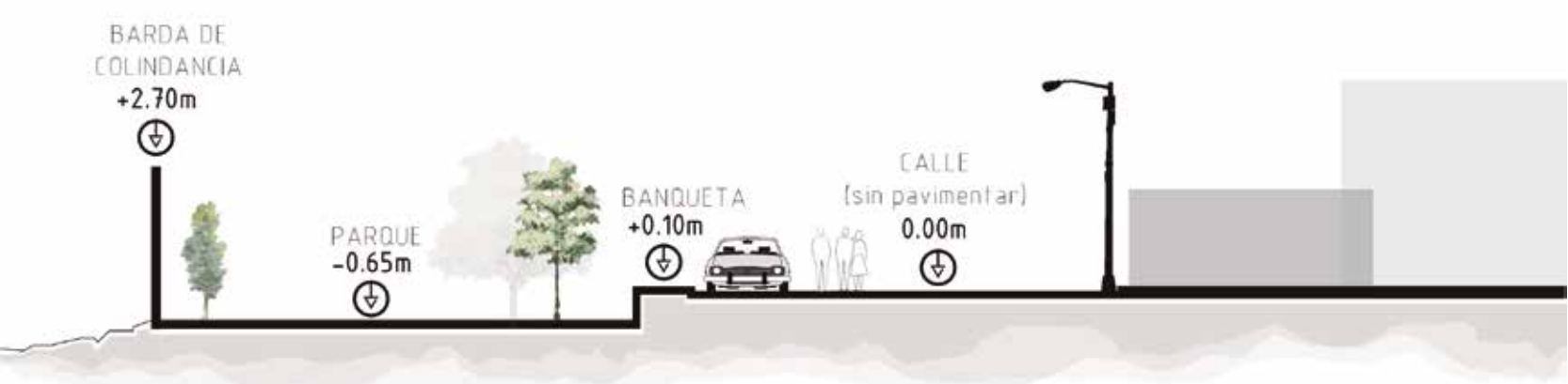
Figura 6.7.2 Levantamiento del terreno del parque, con medidas y mobiliario existente
