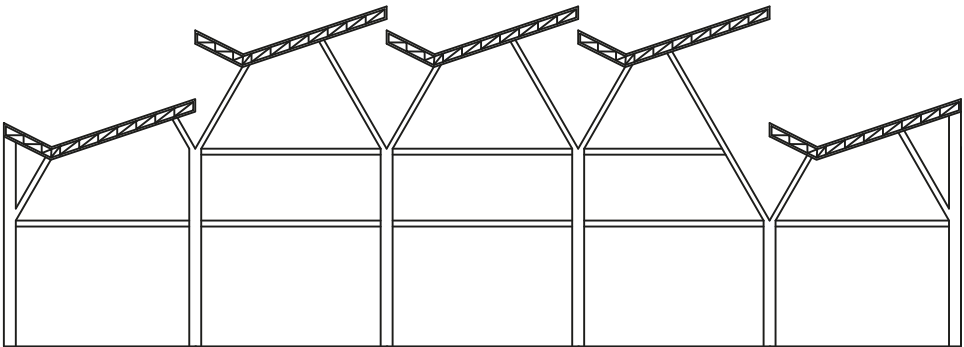
Figura 8.2.2: Boceto en corte de la cubierta de la propuesta 2
