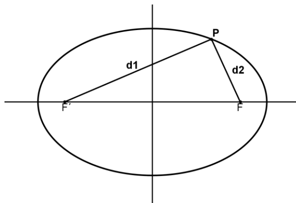
Figura geométrica de la Elipse ( d_1 + d_2 = \text{constante} )
