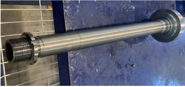
Fig. 12. Eje maquinado en torno sin perforaciones.
