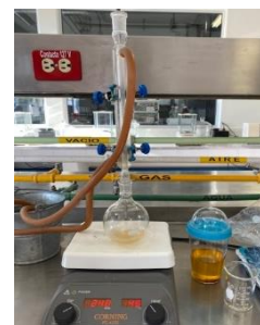
Fig. 2: Proceso de saponificación de aceite de cocina usado durante calentamiento en sistema de reflujo. Elaboración propia (2023).
