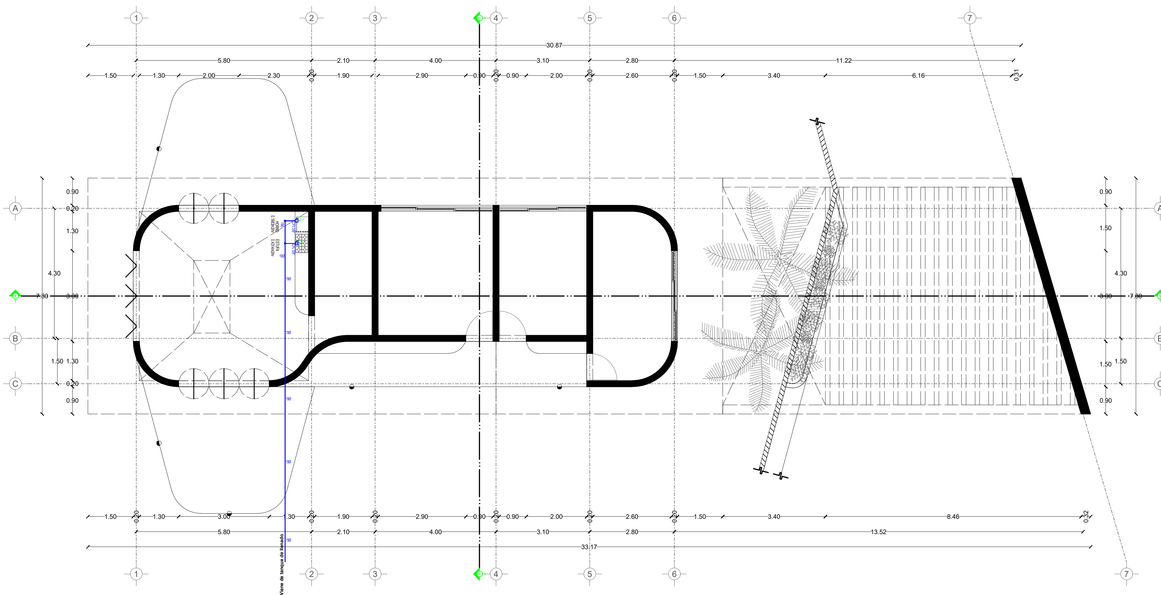
Planta Módulo de cafetería y consultorios
