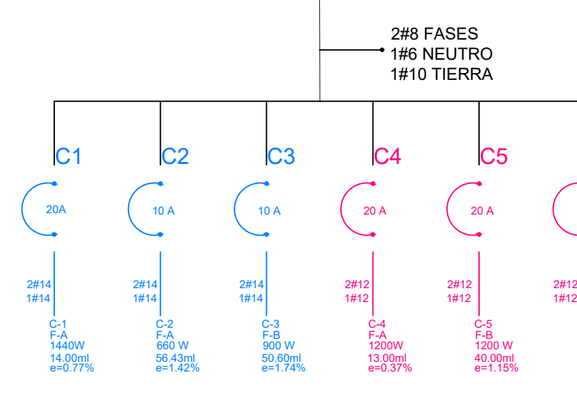
Diagrama unifilar Módulo Canoterapia Tubo verde de 21mm 2X40A
