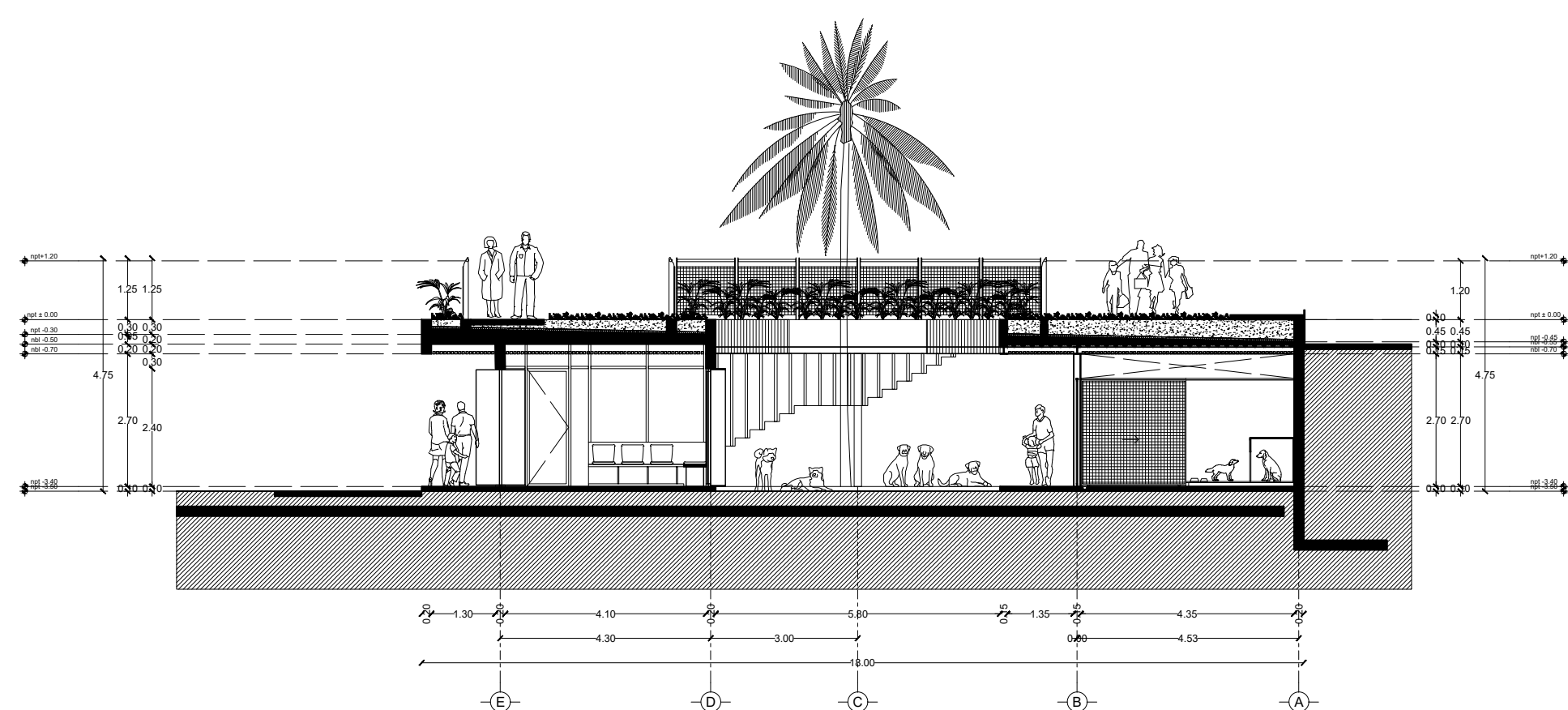
Corte Y-Y'
