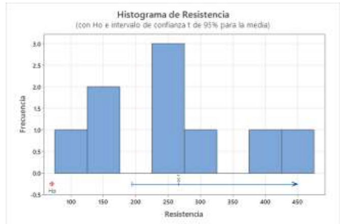
Fig. 4: Histograma.
