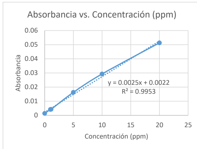
Fig. 18. Curva de calibración del Pb. Fuente: Elaboración propia.
