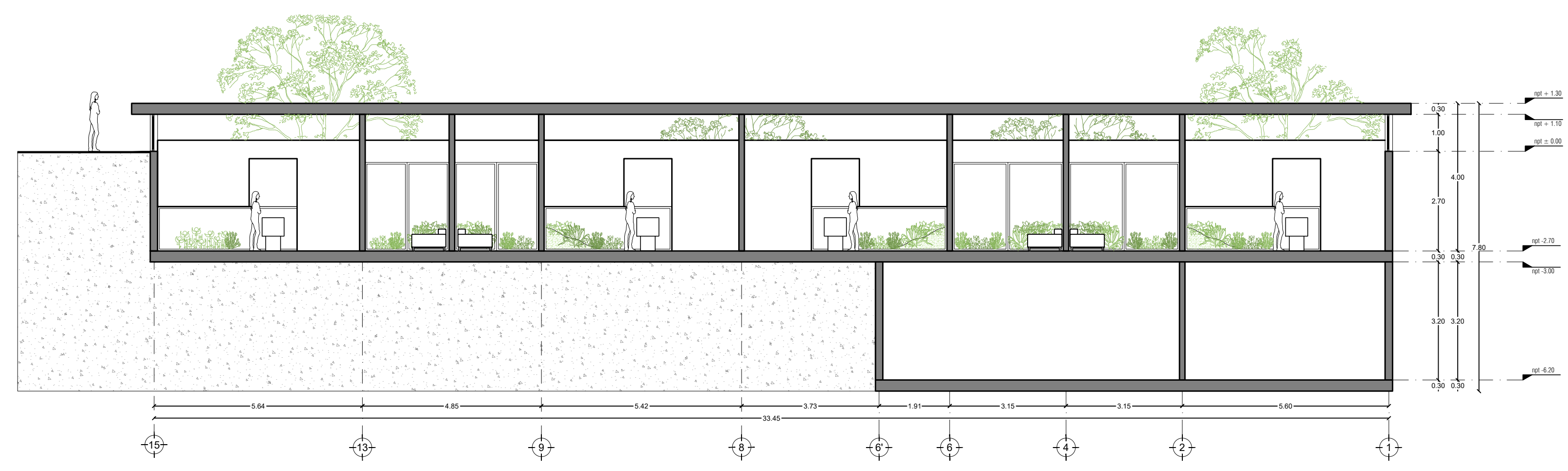
CORTE 04 - X-X'
