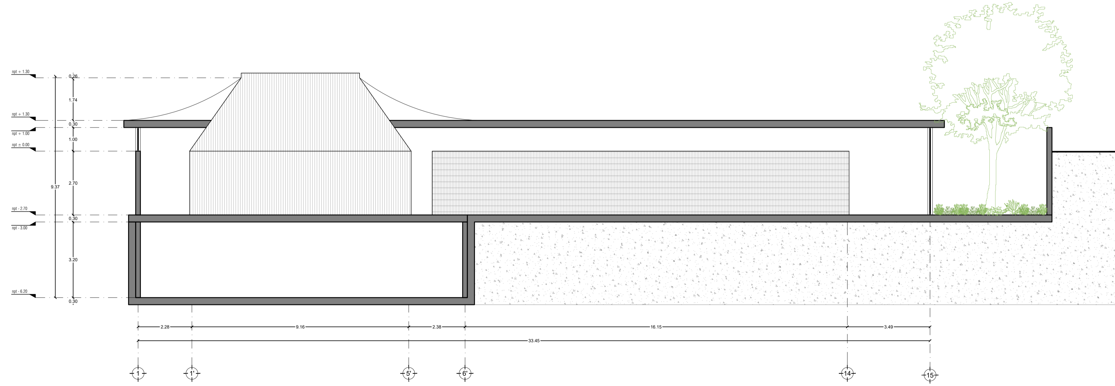
CORTE 06 - Z-Z'
