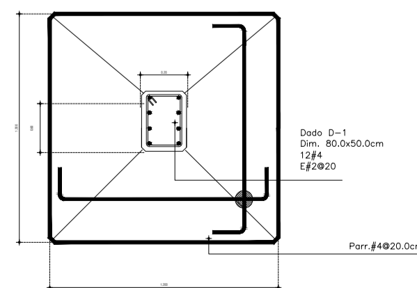
Detalle de Zapata Z-1
