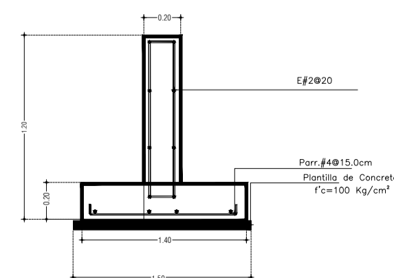
Detalle de Zapata Corrida ZC-1
