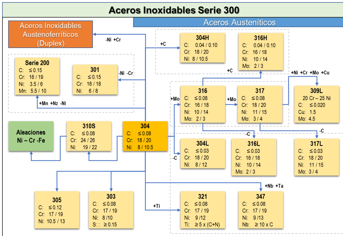
Figura 9. Aceros Austeníticos [11]
