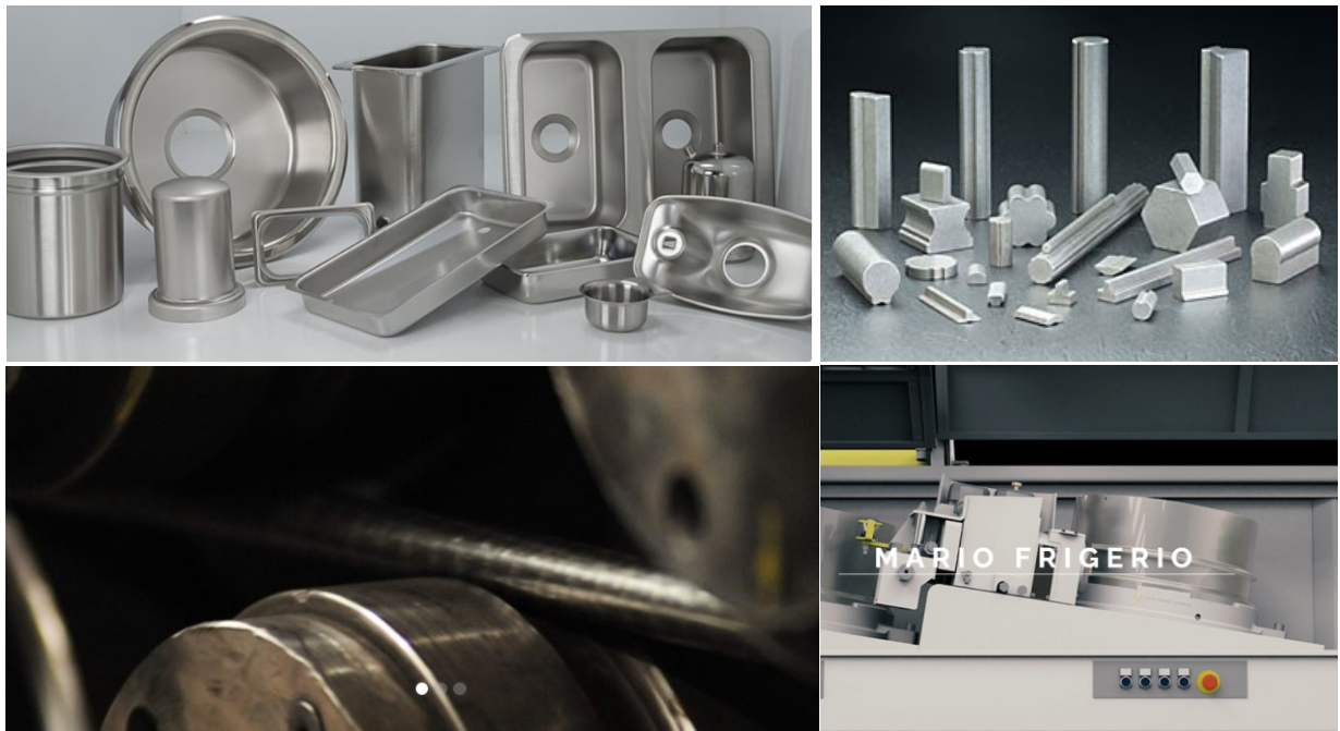
Figura 14. Proceso de formado: partes formadas mediante un embutido profundo e hidro formado [34], perfiles con formas especiales fabricados mediante extruido en frío [35], formado en frío de una barra [36], sección de una máquina para trefilado de alambre [37]
