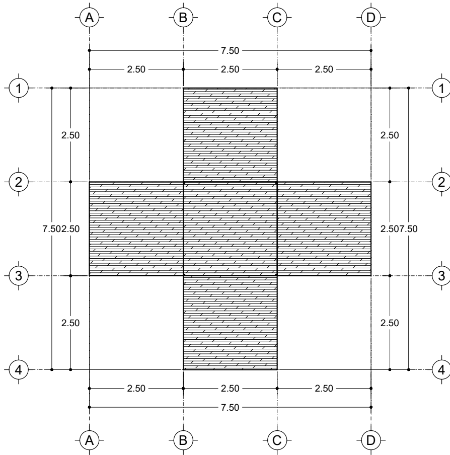
Planta de Cubiertas (abierta)
