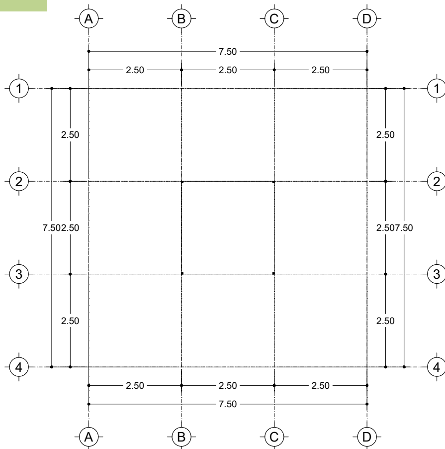
Planta Arquitectónica
