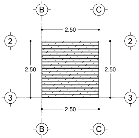
Planta de Cubierta (cerrada)
