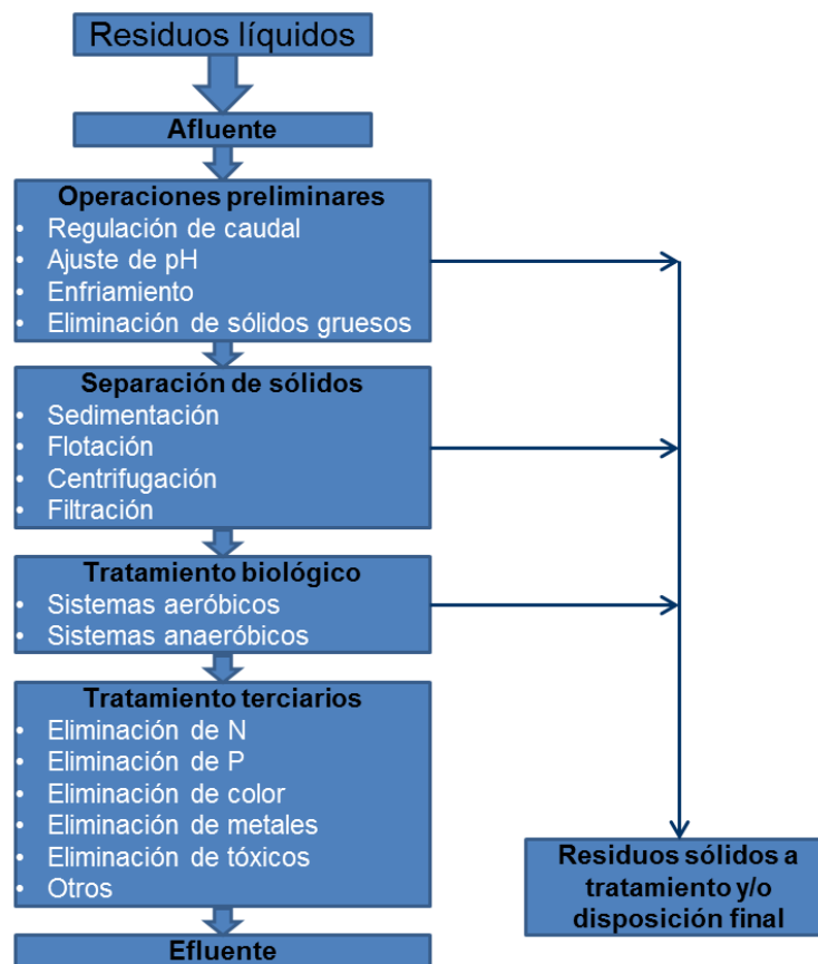
Figura 10. Sistema de tratamiento de residuos líquidos.
