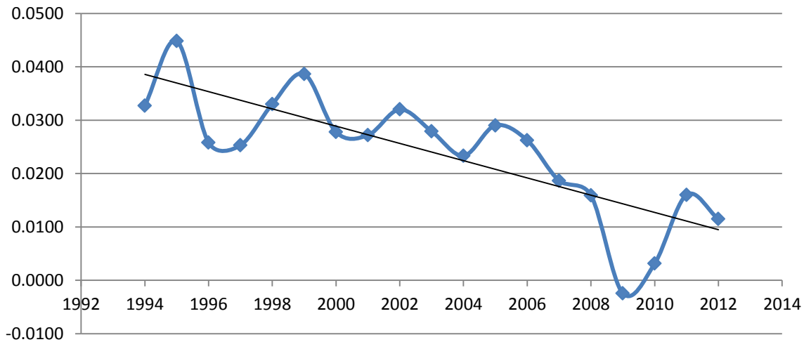
Gráfica 4.5. Productividad Total de los Factores 1994-2012
