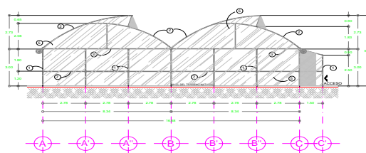
ALZADO FRONTAL ESC. 1 : 100
