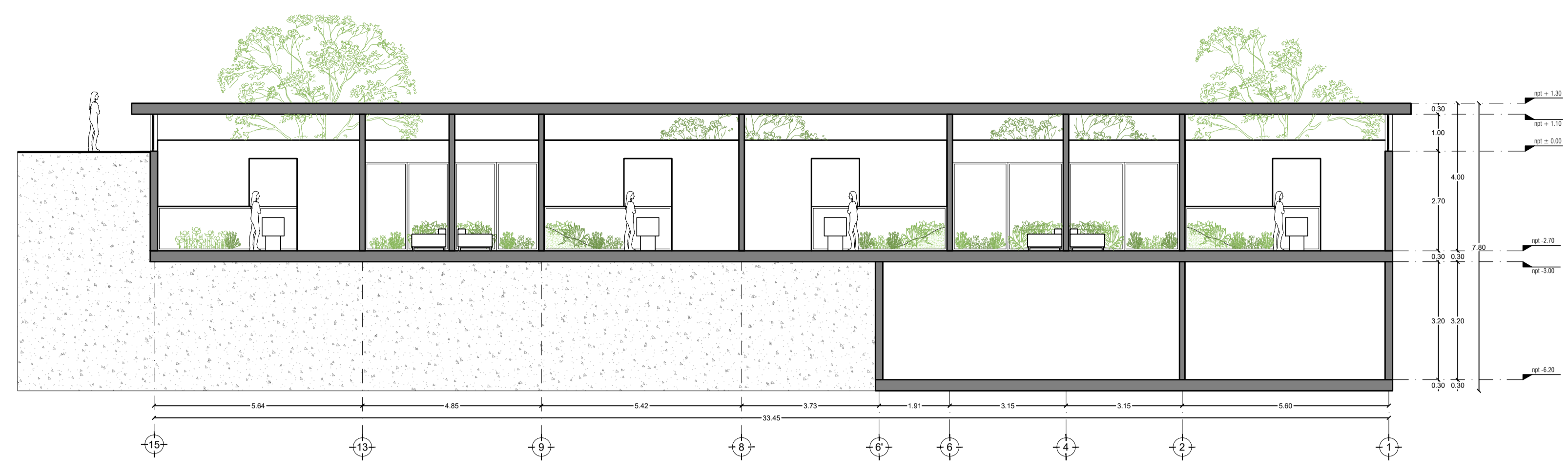
CORTE 04 - X-X'
