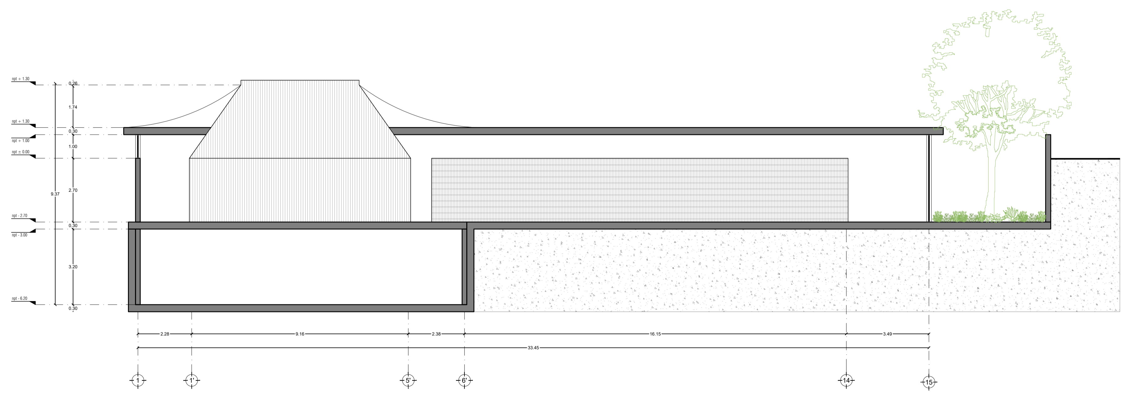
CORTE 06 - Z-Z'
